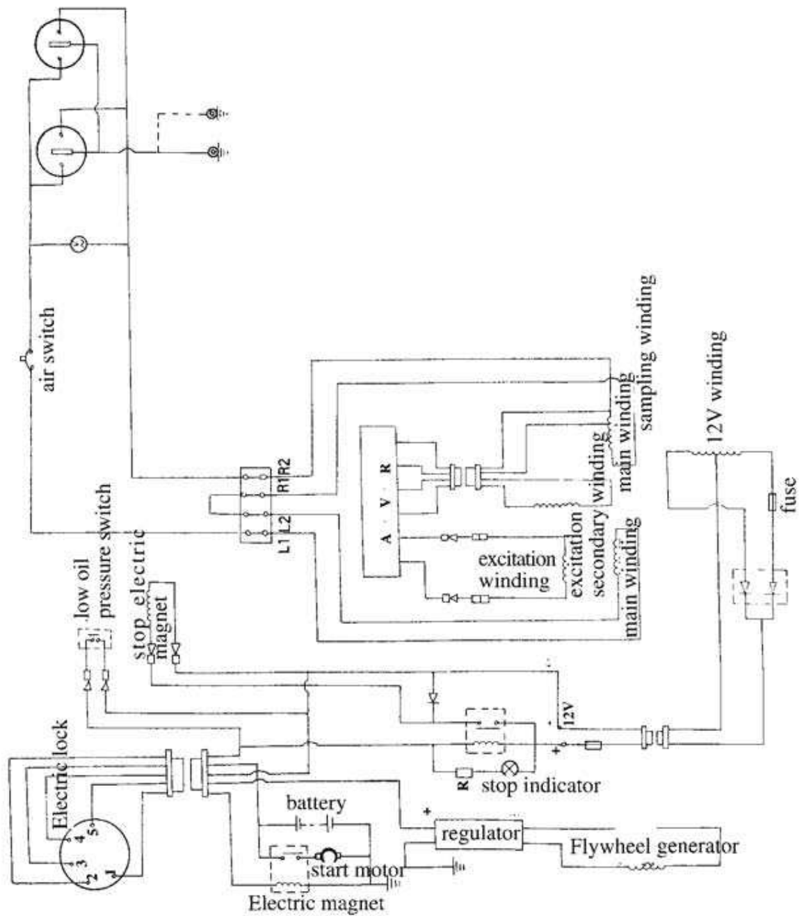
12.13 KDE2200E/KDE3500E/KDE5000E Sähköinen kaavio (yhdeällä jänniteulostulolla)
