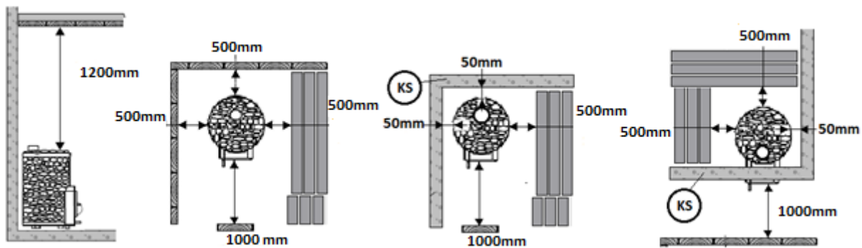
Kuva 3. Suojaetäisyydet
